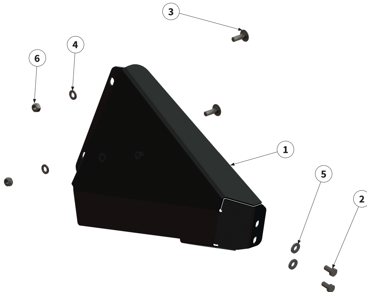
SEITENABWEISER | Side deflector | Déflecteur latéral | Deflector lateral |
